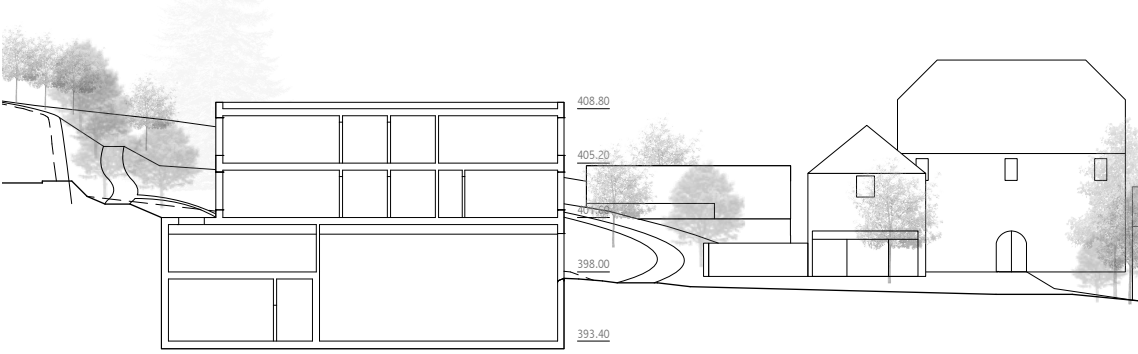
Coupe B-B
